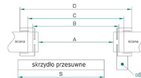
system przesuwny naścienny z zabudową
