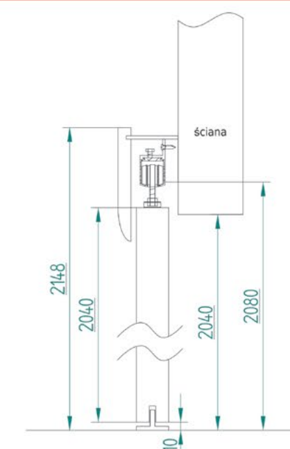
system przesuwny naścienny bez zabudowy
