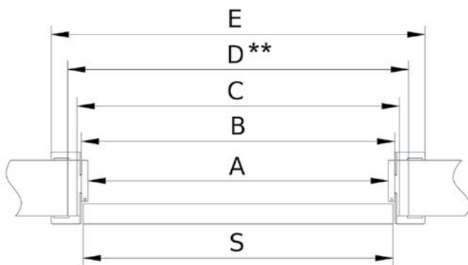
Wymiary (szerokość) ościeżnic panelowych regulowanych bezprzylgowych (OPB)
