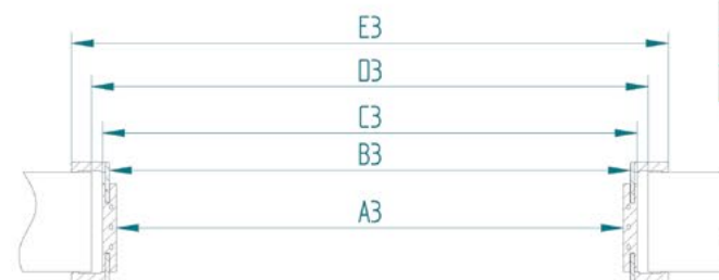
Tunel Regulowany (TR)(dawniej TPP)
