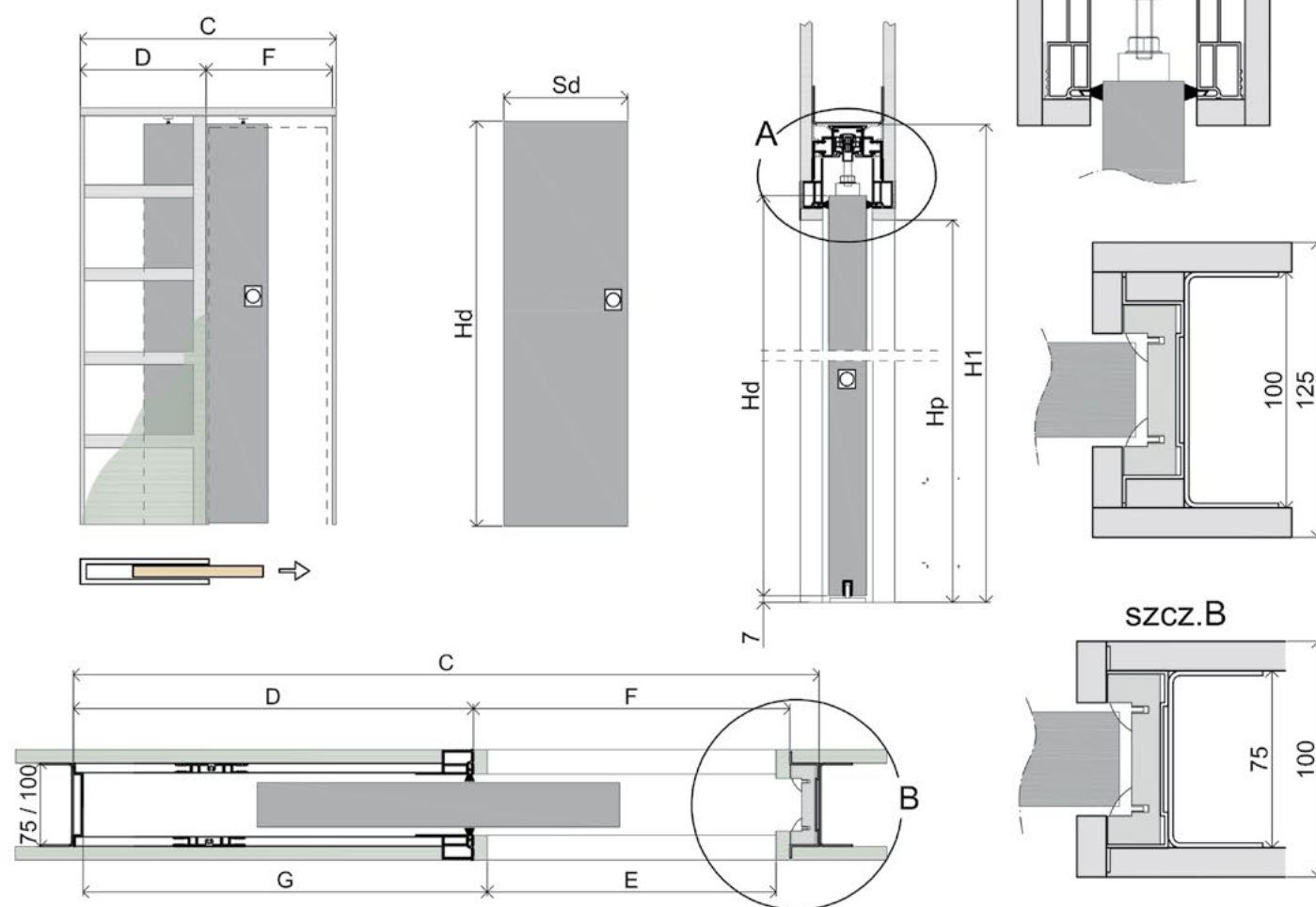
Kaseta Bezościeżnicowa B15 1190,00 zł netto/1463,70 zł brutto
