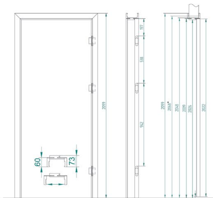
Zakresy ościeżnic panelowych regulowanych bezprzylgowych (OPB)
