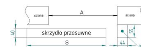
system przesuwny naścienny bez zabudowy
