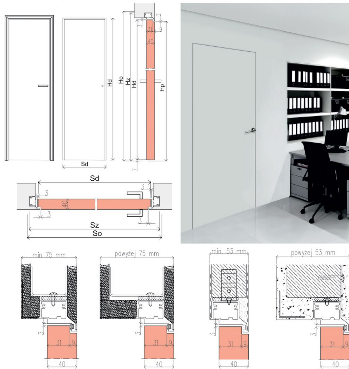
wymiary standardowe dla drzwi przylgowych otwieranych do wewnątrz
