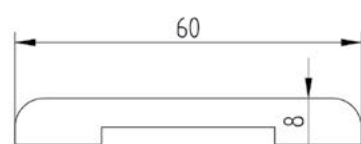
PRZEKRÓJ OPASKI MASKUJĄCEJ
